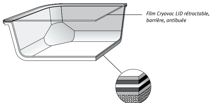
Barquette barrière Cryovac Vitembal en polystyrène expansé, avec protection coextrudée barrière de Cryovac
